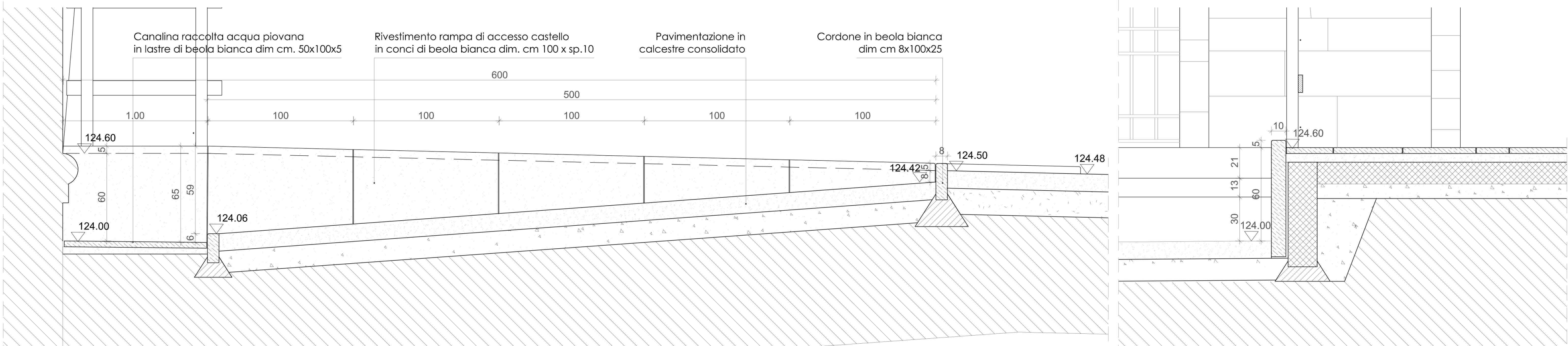
PARTICOLARE RAMPA DI ACCESSO AL CASTELLO - SEZIONE E-E - Scala 1:20
