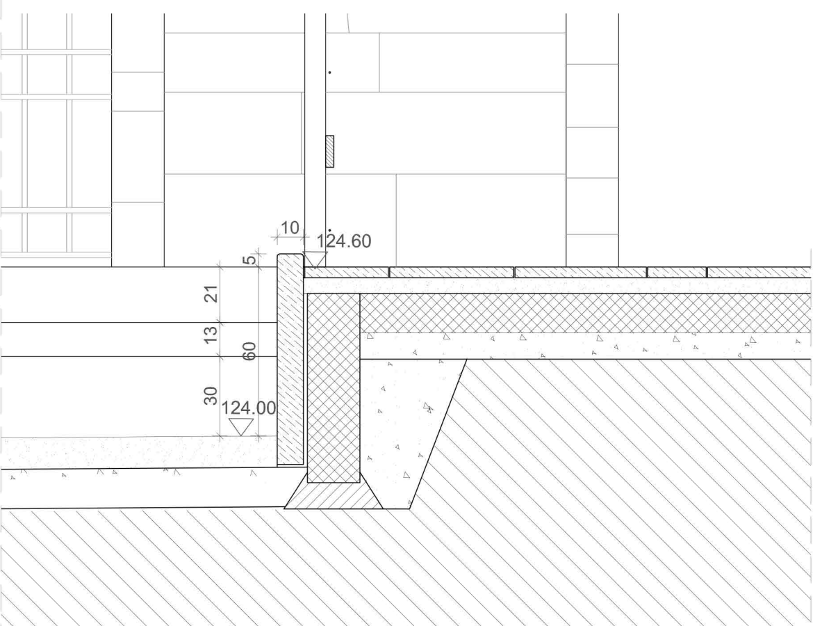
SEZIONE D-D - PARTICOLARE - Scala 1:20
