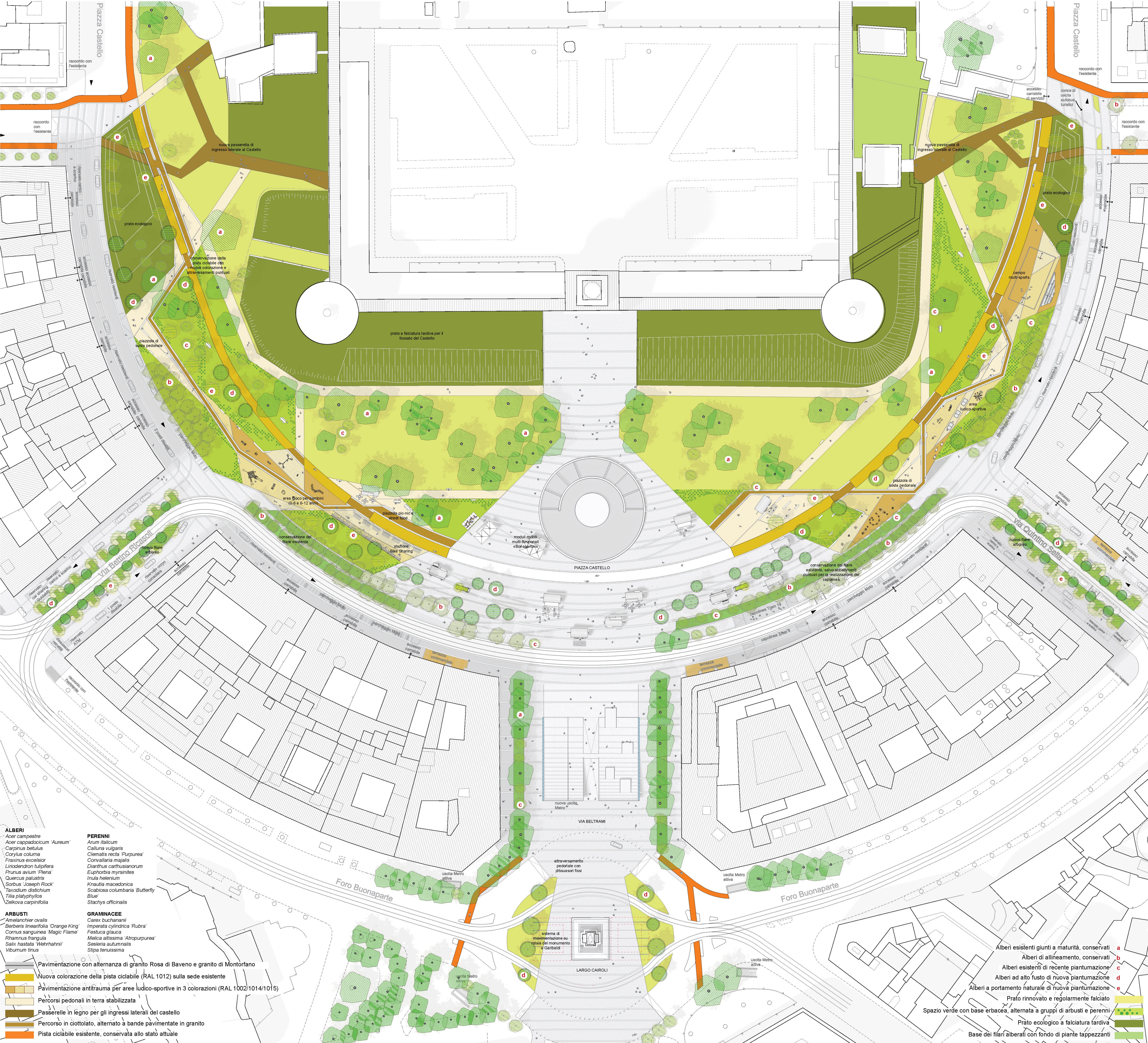
PLANIMETRIA GENERALE_SCALA 1:500
